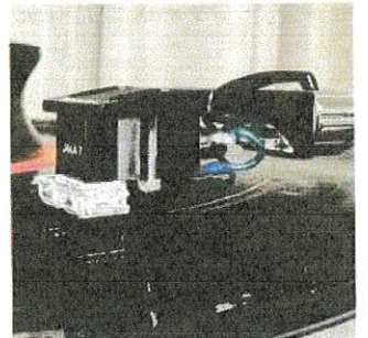
使用カートリッジJICO「J44A 7 IMP NUDE」+テクニクス製ヘッドシェル。交換計は「N44-7」(無振丸針、針圧1.5~3.0g)
